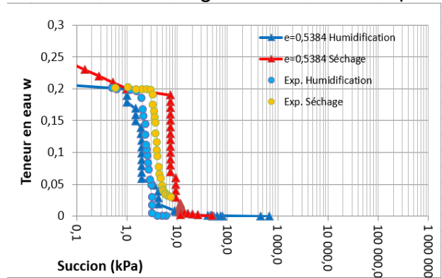
Figure 3 Courbe de rétention pour le chemin de séchage et de mouillage - sable de Fontainebleau NE1-1
