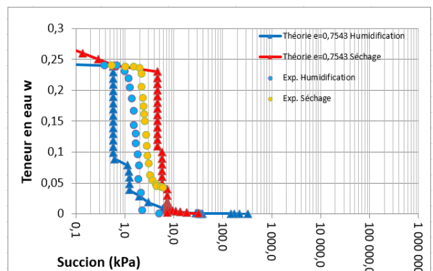
Figure 7 Courbe de rétention pour le chemin de séchage et de mouillage - sable Hostun HNI
