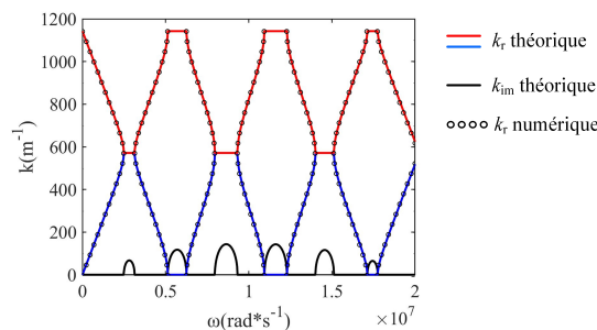
FIGURE 3 – Comparaison des solutions analytiques et numériques de la structure 1D
