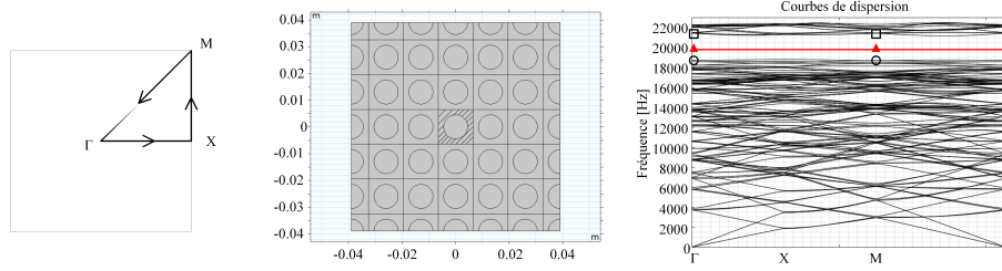
FIGURE 10 – Modèle multicellulaire 6L \times 6L avec un défaut en module d'Young de la matrice de la cellule centrale et les courbes de dispersion avec le mode localisé marqué en rouge
