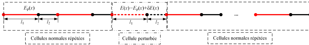
FIGURE 6 – Modèle multicellulaire de 12 cellules avec un défaut introduit sur une cellule en perturbant le module d’Young
