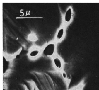
Figure 1 – UO 2 irradié présentant des bulles intergranulaires [1].
