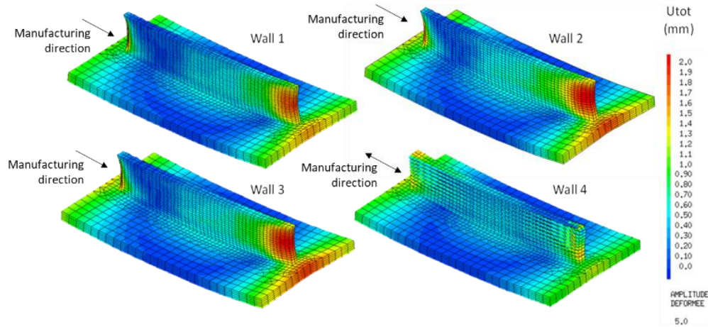
Figure 8 – Comparaisons des champs de déplacement sur le maillage déformé (amplifié 5 fois) pour les quatre murs réalisés. Le code couleur représente l'intensité du déplacement total, sans amplification.
