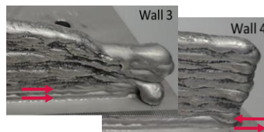
Figure 2 – Différents types de pièces fabriquées en acier inoxydable 316L avec le procédé TIG-WAAM.
