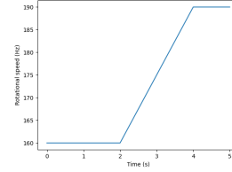
(d) Rotational speed profile
