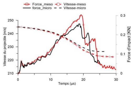
Figure 8 – Évolutions des vitesses du projectile et des forces d'impact : comparaison des modélisations méso et micro (multi-échelle).
