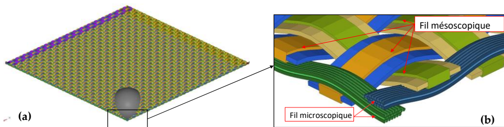
Figure 7 – Modèle multi-échelle méso-micro d'un tissu 2D avec des éléments coques.
