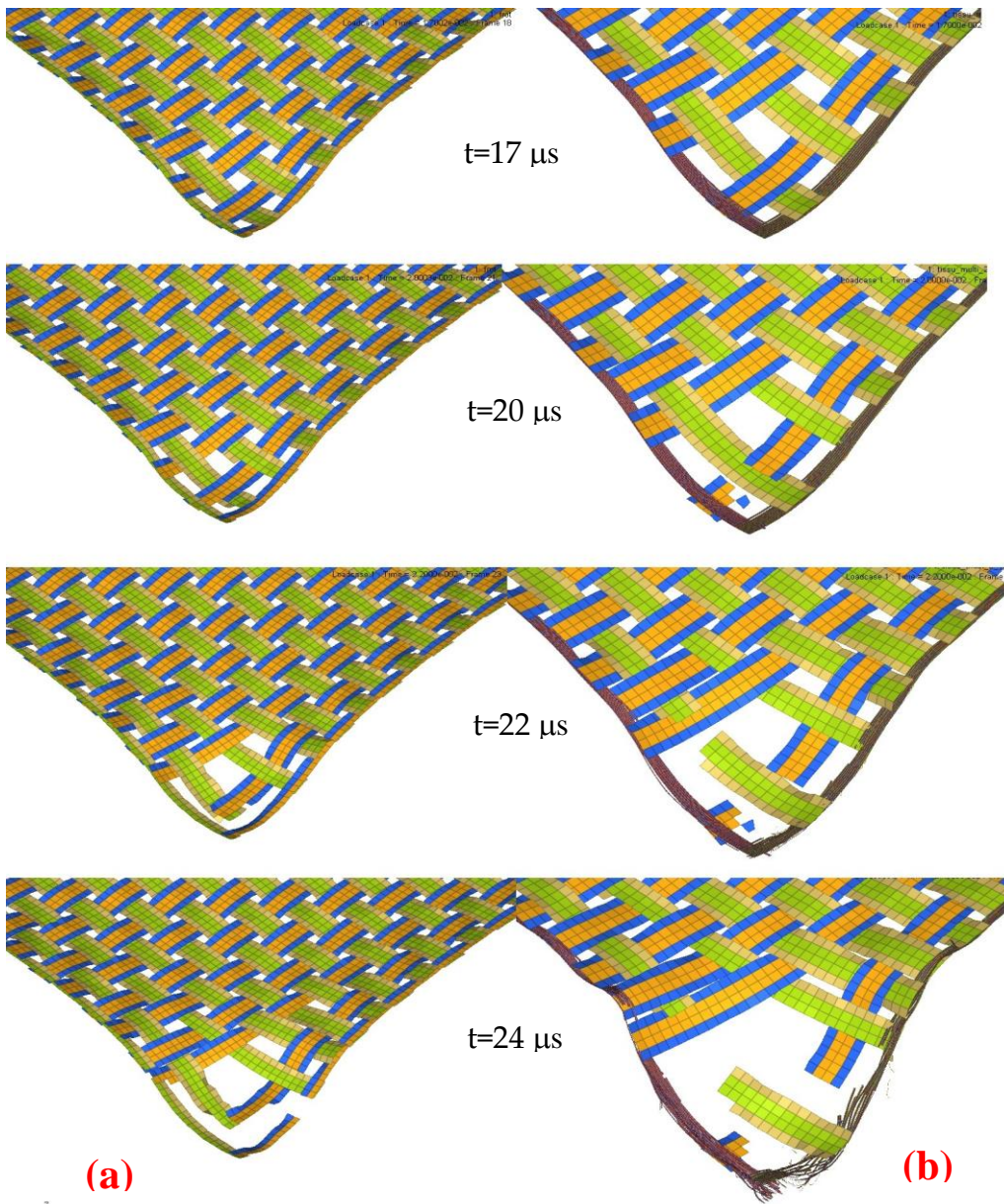
Figure 9 – Comparaison l'état d'endommagement du tissu à la zone d'impact à différents instants : (a) Modèle mésoscopique ; (b) Modèle microscopique.
