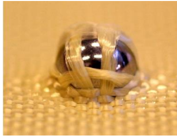
Figure 1 – Détails de la zone d’impact d’un tissu Kevlar KM2 (vue face arrière du tissu) [7].
