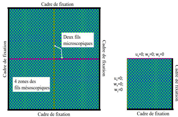
Figure 6 – Conditions aux limites de la modélisation microscopique : (a) Modèle complet ; (b) Quart du modèle.
