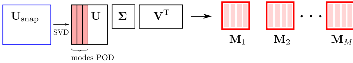
FIGURE 4 – Génération des bases de matrices réduites à partir d’une SVD.
