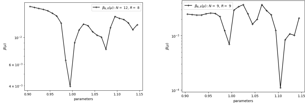
FIGURE 4 – Construction standard : \beta_{N,R}(\mu) . Gauche : (N,R) = (12,8) . Droite : (N,R) = (9,9) .
