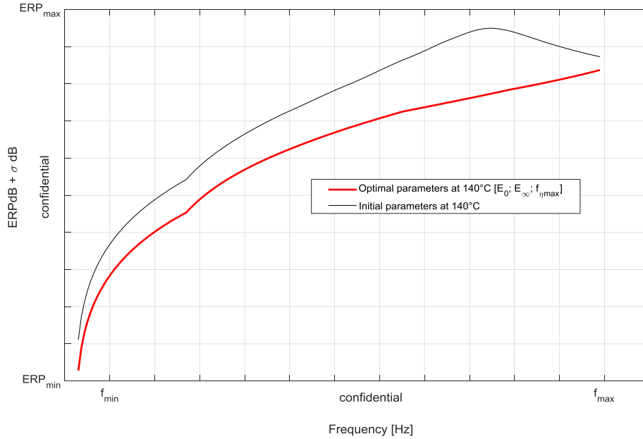
Figure 2: ERP du moteur électrique en fonction de la fréquence avant et après optimisation du comportement viscoélastique de la résine d'enrobage à 140°C
