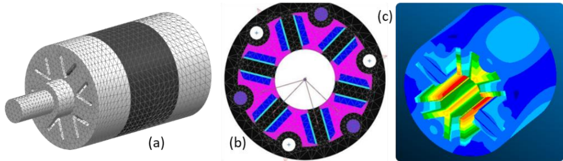
Figure 1: MEF du moteur électrique (a), vue en coupe avec la résine d'enrobage (rose) (b), mode de vibration (2,0) (c)
