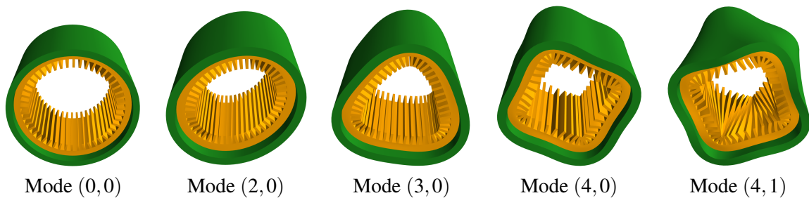
FIGURE 4 – Exemple de déformées modales du modèle standard de Rayleigh-Ritz.
