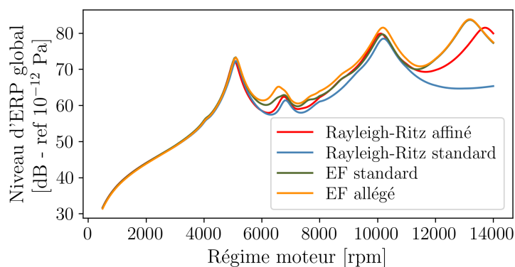
FIGURE 5 – Comparaison des niveaux d'ERP estimés par les modèles de Rayleigh-Ritz et les modèles EF.
