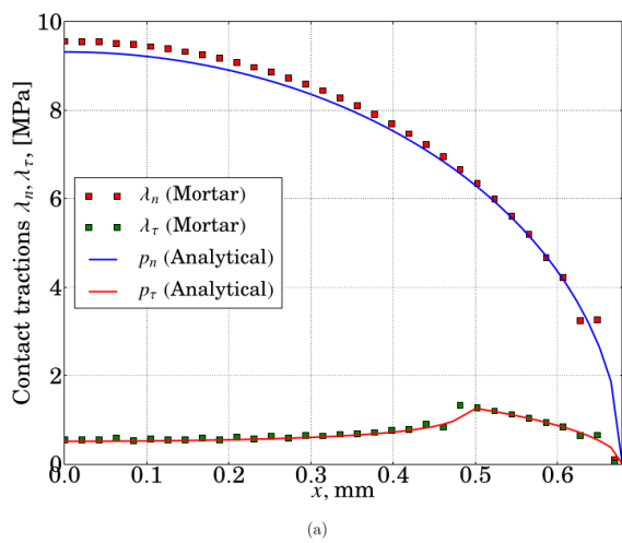
FIGURE 5 – Vecteur-contrainte normal et tangentiel dans l’interface de contact (a) mortier classique, (b) MorteX.
