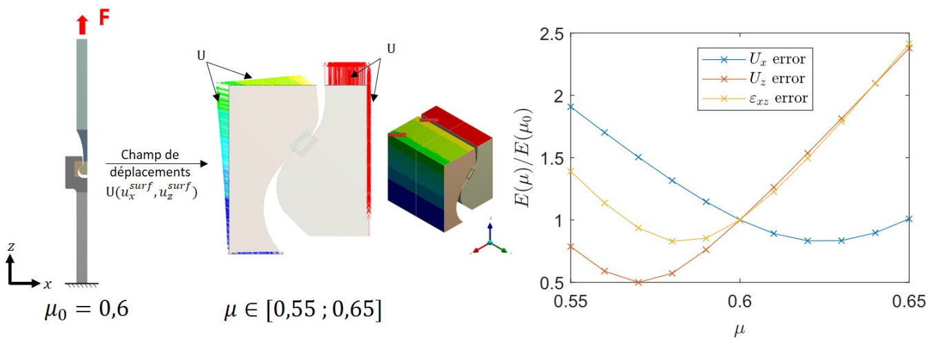
FIGURE 5 – Schéma de principe du second sous-modèle avec l’hypothèse sur les conditions aux limites. Tracé de l’erreur associée en fonction du coefficient de frottement
