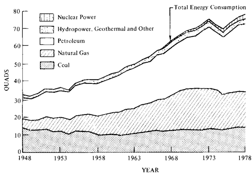
Figure 8. Représentation classique de l'évolution du mix énergétique énergétique
