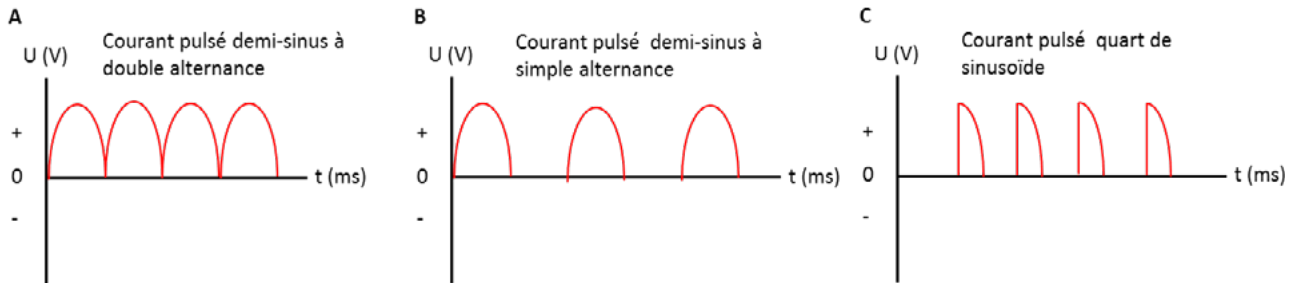
Figure 11. A: profil d'un courant continu pulsé demi-sinus à double alternance.
