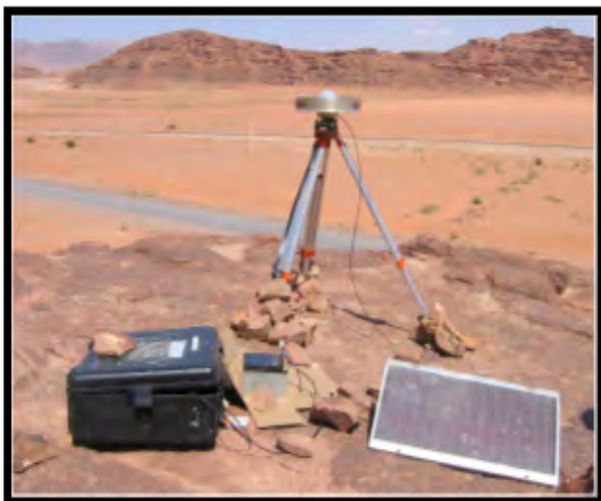
Figure 1: Campagne GPS en Jordanie. (Photographie Yann Klingner).
