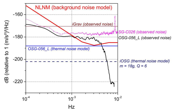
Figure 2. Densités spectrales de puissance de plusieurs types de gravimètres supraconducteurs (à noter la réduction prévue du bruit instrumental de l'iOSG par rapport au meilleur gravimètre actuel (OSG-056_L) en fonctionnement à BFO en Allemagne. Le niveau de bruit (instrumental + environnemental) actuel à l'Observatoire Gravimétrique de Strasbourg est représenté en rose (SG-C026).
