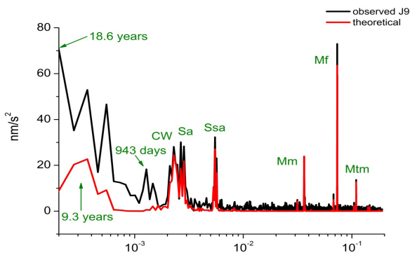
Figure 1. Spectres d'amplitude prédits et observés associés aux variations temporelles de gravité observées à Strasbourg de 1987 à 2014. Les principales ondes de marées longue-période ainsi que l'oscillation de Chandler (CW) sont indiquées.
