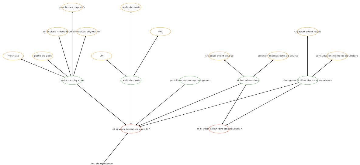
Figure 1 : Modélisation d'un réseau Bayésien - l'exemple de la dénutrition.
