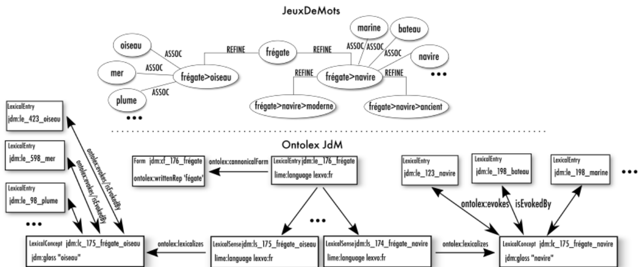
FIGURE 4 – Un exemple de la conversion des nœuds de termes et des raffinements vers le modèle Ontolex pour le terme « frégate » (Figure 1 de Tchechmedjiev et al. (2017)).
