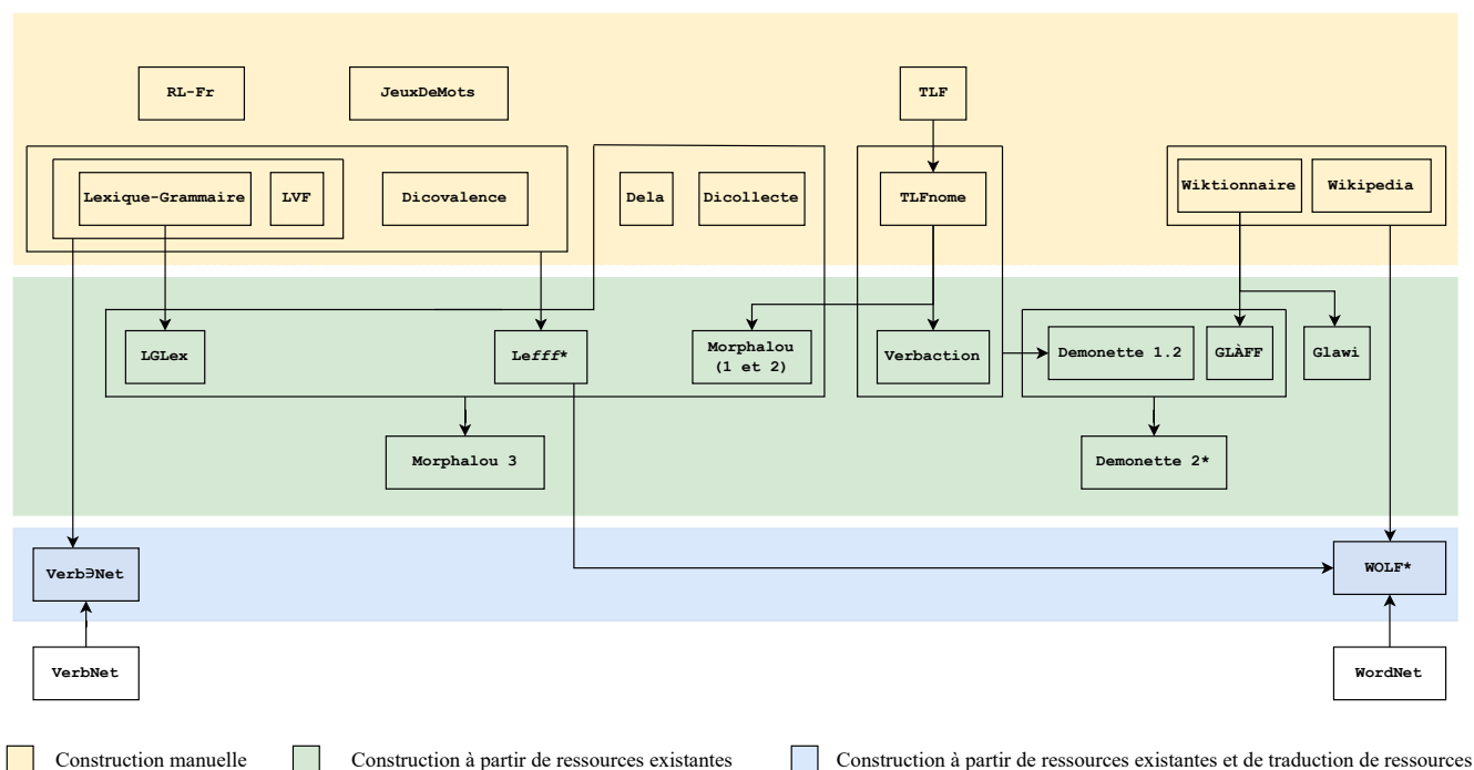
FIGURE 3 – Ressources lexicales du français créées à partir de ressources existantes (les ressources suivies d’un astérisque ont été créées avec d’autres ressources supplémentaires qui ne figurent pas sur ce schéma.).
