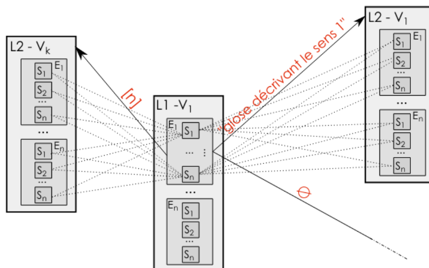
FIGURE 5 – Les données de DBnary post-extraction sans pré-traitement des relations de traductions (Figure 4.1 de Tchechmedjiev (2016)).
