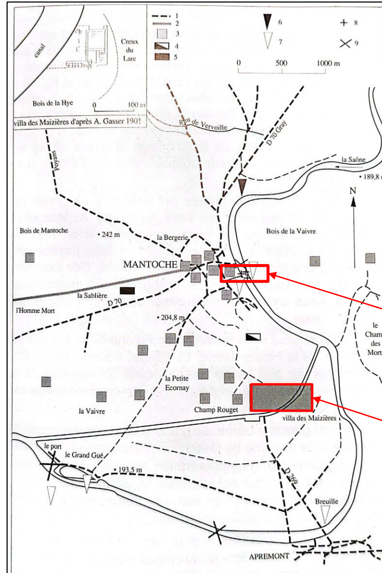
fig. 26. Mantoche : plan d'ensemble des vestiges (d'après S. Labre 1986, complété par M. Demesy et N. Bonvalot, 1992). 1. axe moderne ; 2. voie romaine non confirmée ; 3. vestiges antiques ; 4. inhumation ; 5. incinération ; 6. atelier céramique ; 7. mobilier céramique ; 8. monnaie ; 9. gué.
