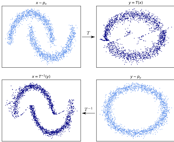
FIGURE 1 – Résultats obtenus lorsque la distribution cible p_X est une double-lune (en haut à gauche) et la distribution de base p_Y est un cercle (en bas à droite).
