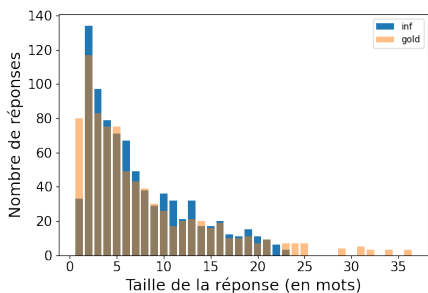
(a) basic-Frame-ctx
