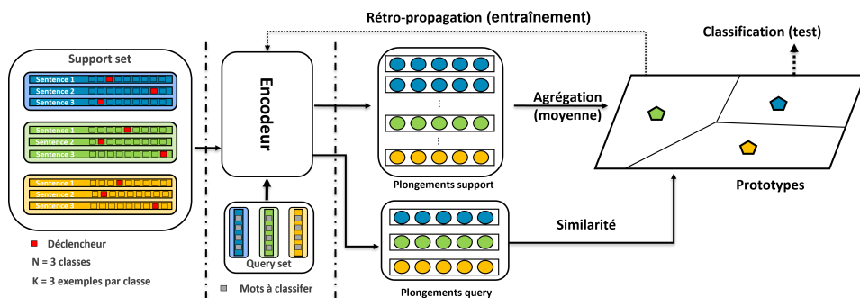
FIGURE 1 – Vue d’ensemble du modèle
