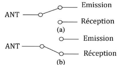
Figure 1. Représentations idéales d'un switch SPDT. (a) à l'état OFF. (b) à l'état ON.
