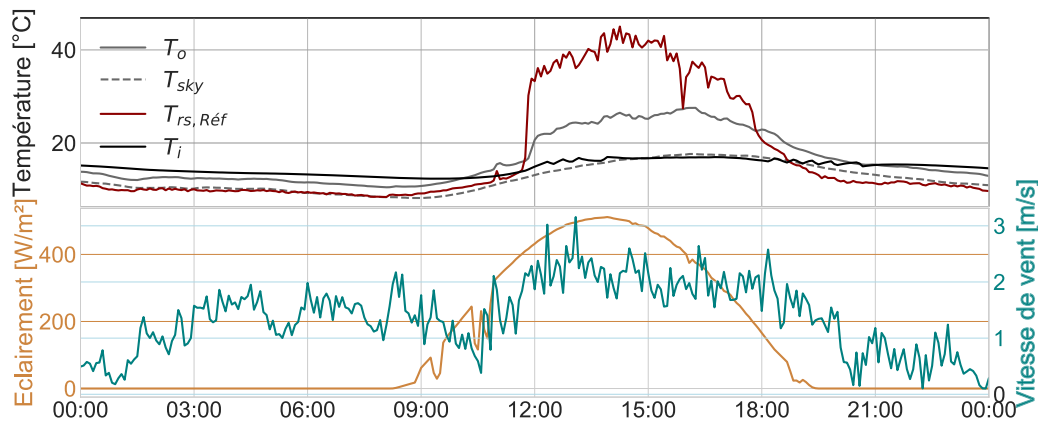
Figure 3 : Evolution des conditions météorologiques ( T_{sky} , T_o , E , v ), de la température intérieure du caisson ( T_i ) et de la température de la surface de la toiture de référence ( T_{rs, Réf} ) – le 9/10/2021 à La Rochelle
