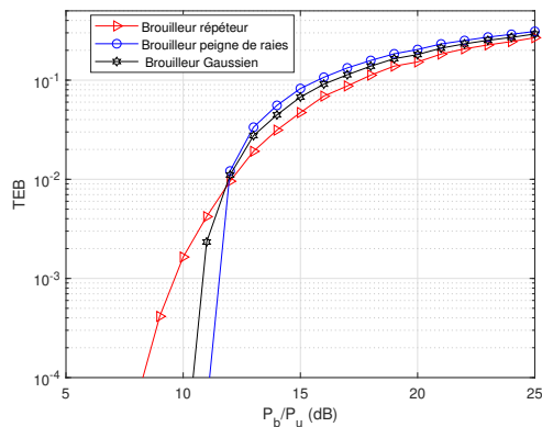
FIGURE 5 – TEB avec BPSK tournée (2ème scénario).
