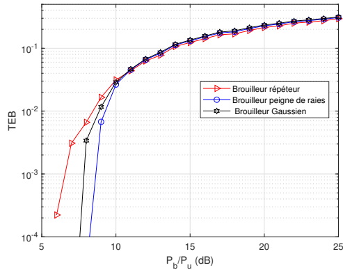
FIGURE 4 – TEB avec BPSK conventionnelle (2ème scénario).
