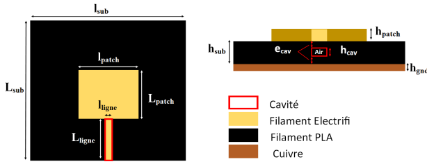
Figure 3. Dimensions de l'antenne patch et de la cavité
