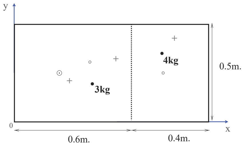
Figure 2. Géométrie de la structure \Omega . • masses concentrées, + ressorts, ⊙ point d'excitation, ○ points d'observation.
