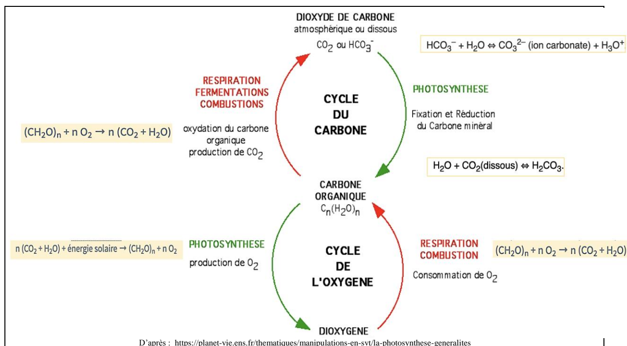
Schéma 5: Les mécanismes de la photosynthèse générale
