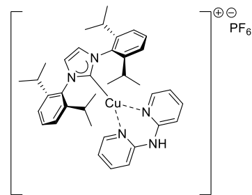
Fig. 2 [Cu(IPr)(dpa)][PF 6 ].
