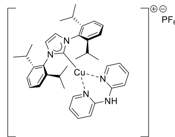
Fig. 2 [Cu(IPr)(dpa)][PF 6 ].
