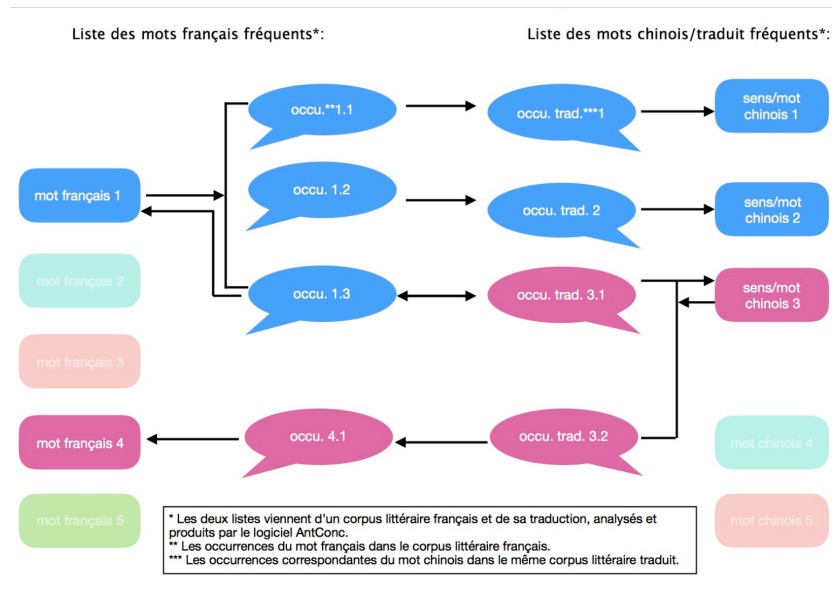
FIGURE 2 – Schéma cognitif
