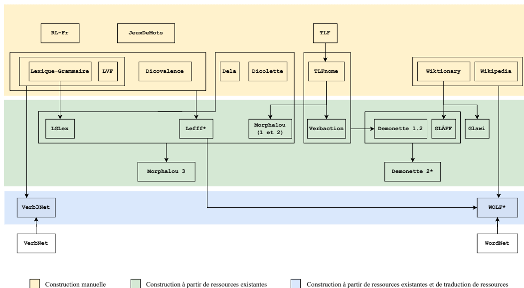
FIGURE 3 – Ressources lexicales du français créées à partir de ressources existantes (les ressources suivies d’un astérisque ont été créées avec d’autres ressources supplémentaires qui ne figurent pas sur ce schéma.).
