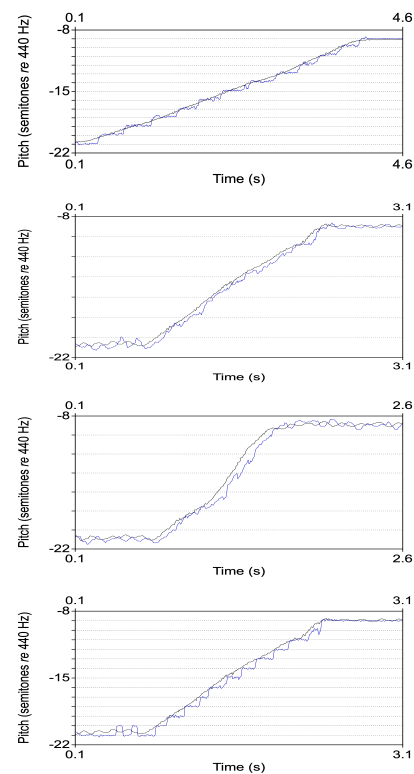
FIGURE 4 – De haut en le bas : Glissando sans vibrato de C3 à C4 pendant 400ms. Glissando lent avec vibrato de C3 à C4. Glissando rapide avec vibrato de C3 à C4. Glissando lent avec vibrato de C3 à C4 avec une correction instantanée
