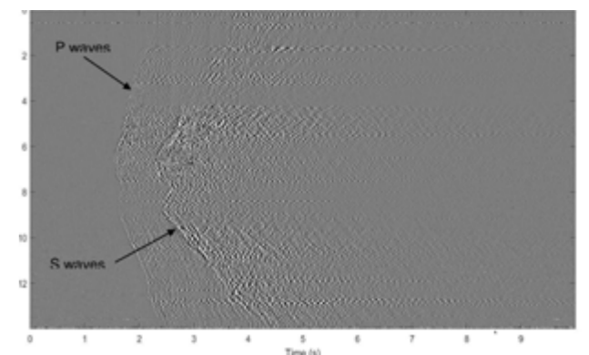
3 - Enregistrement DAS d'une réplique ML=2.0 le 23 novembre 2019, suite au séisme M4.9 du Teil, France. La campagne de mesure s'est faite sur une section de 14km de fibre optique située à proximité immédiate de la zone de rupture. Ces mesures n'auraient pas été possible sans la collaboration du réseau public Ardèche Drôme Numérique, l'opérateur ADTIM et le soutien de la société Febus Optics pour la partie acquisition
