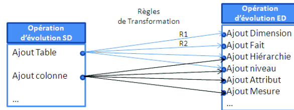
FIG. 5 – Transformation possibles pour les opérations d'ajout de table ou de colonne.
