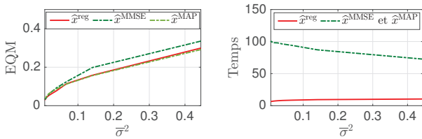
FIGURE 4 – Comparaison avec l’état de l’art. Dans cet exemple \bar{p} = 0.015 et \bar{\sigma}^2 varie. La méthode proposée (rouge) avec |\Lambda^{\text{reg}}| = 500 est comparée aux estimateurs MAP et MMSE bayésiens (vert) obtenus après 10^3 itérations.
