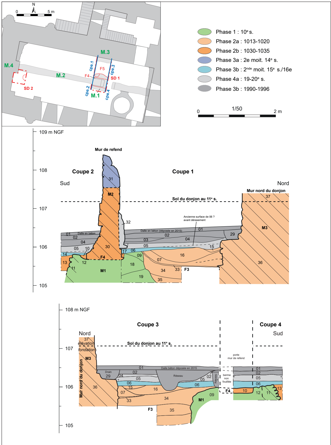
Figure 48 : coupes 1 à 4 du sondage 1
