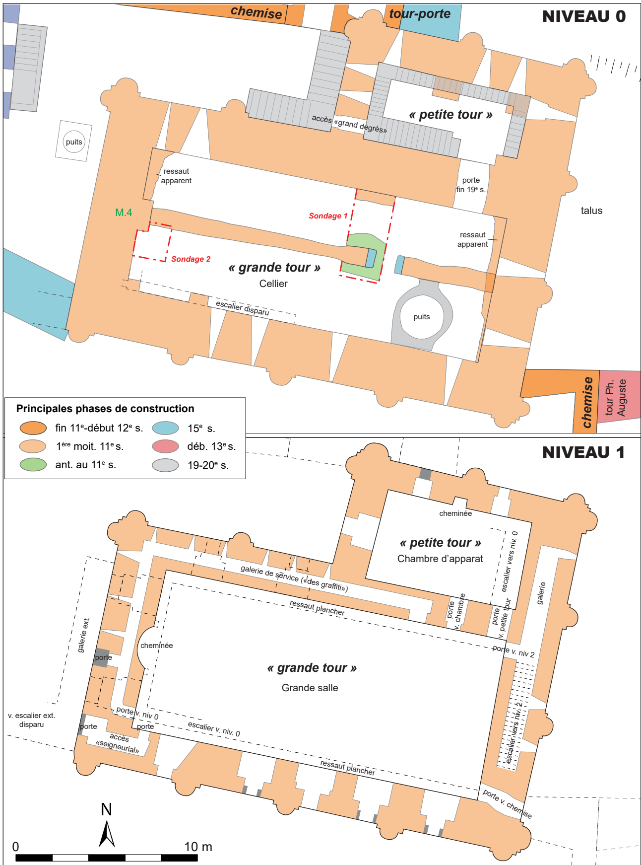
Figure 19 : plans des niveaux 0 et 1 de la tour maîtresse (à partir du relevé 3D de 2017)
