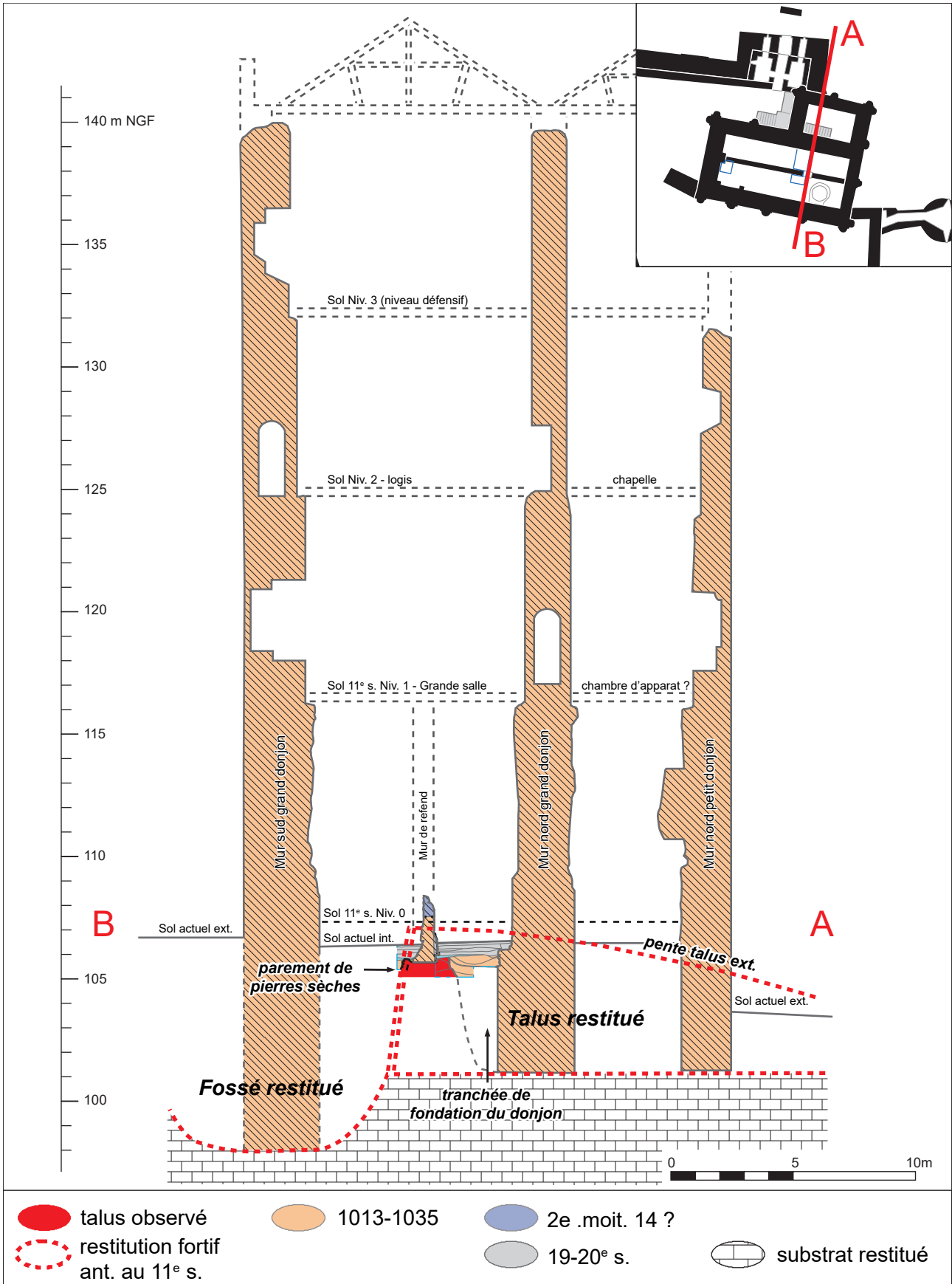
Figure 58 : coupe de la tour maîtresse avec restitution de l'hypothèse d'un rempart de terre et pierre antérieur
