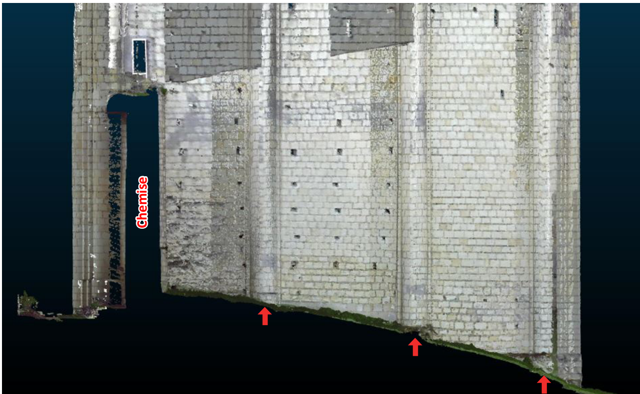
Figure 61 : détail de la face est de la tour maîtresse (issu de la lasergrammetrie, Pellerin 2017), avec le talus de terre et les fondations étagées des contreforts
