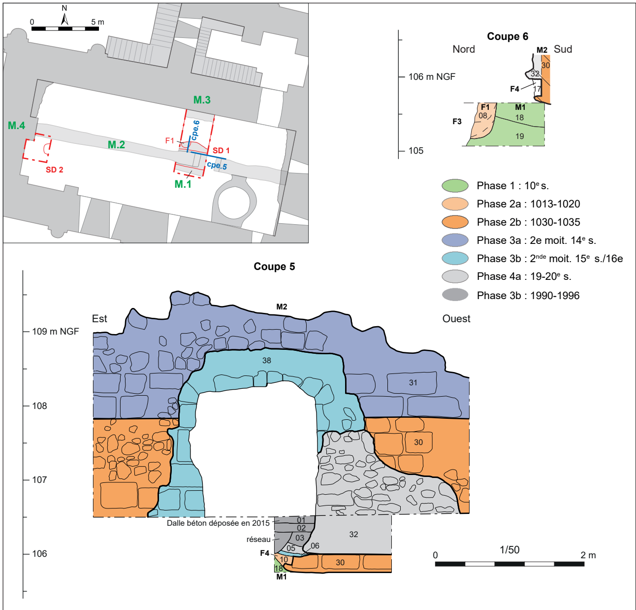
Figure 49 : coupes 5 et 6 du sondage 1
