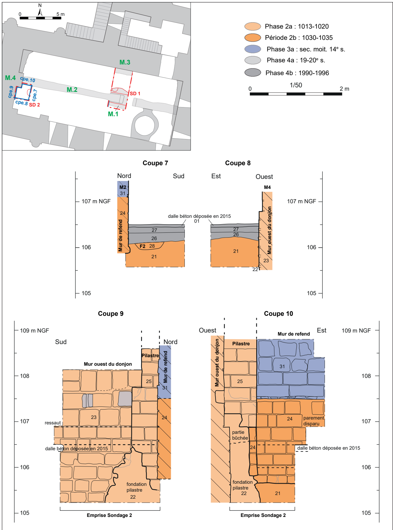
Figure 50 : coupes 7 à 10 du sondage 2
