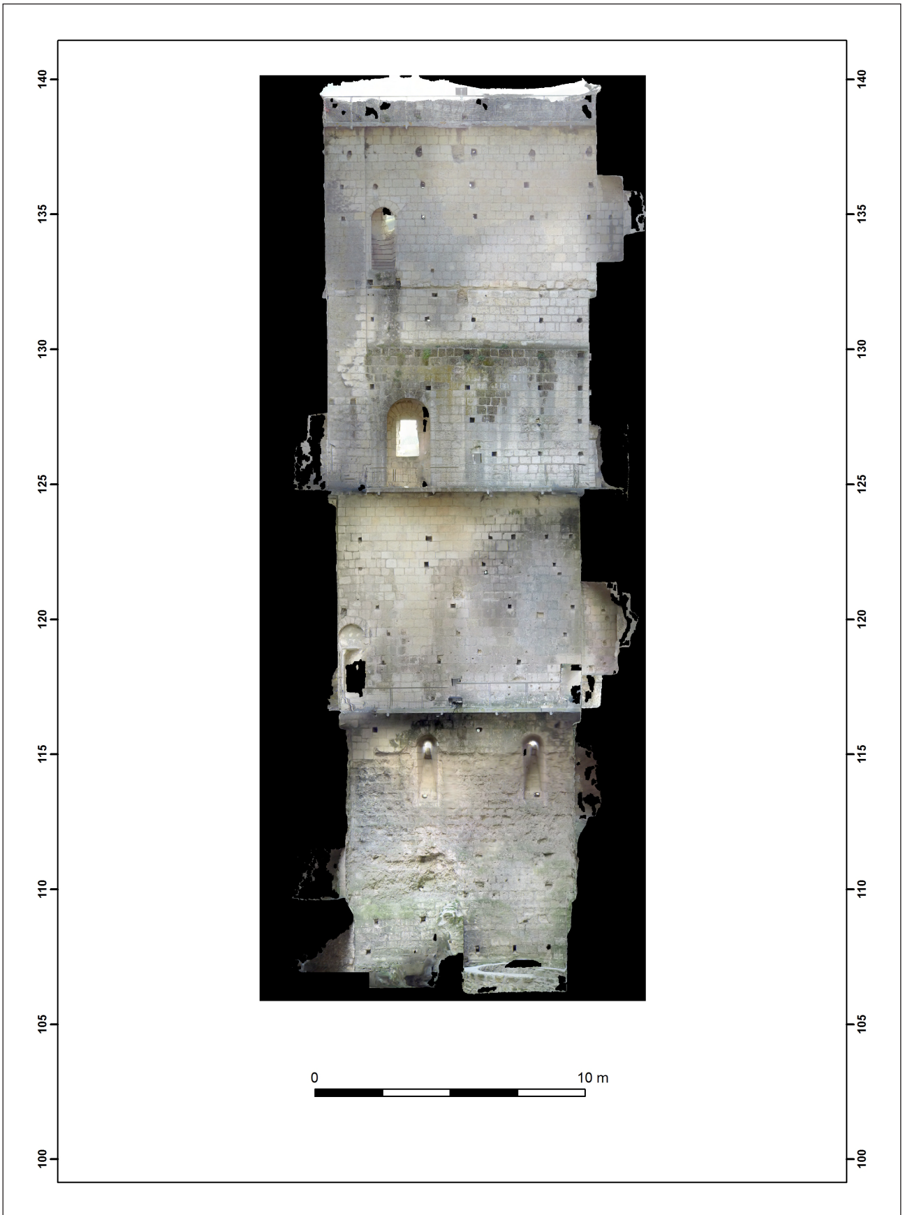
Figure 22 : photogrammètrie de la face interne est de la grande tour (Pellerin 2017)
