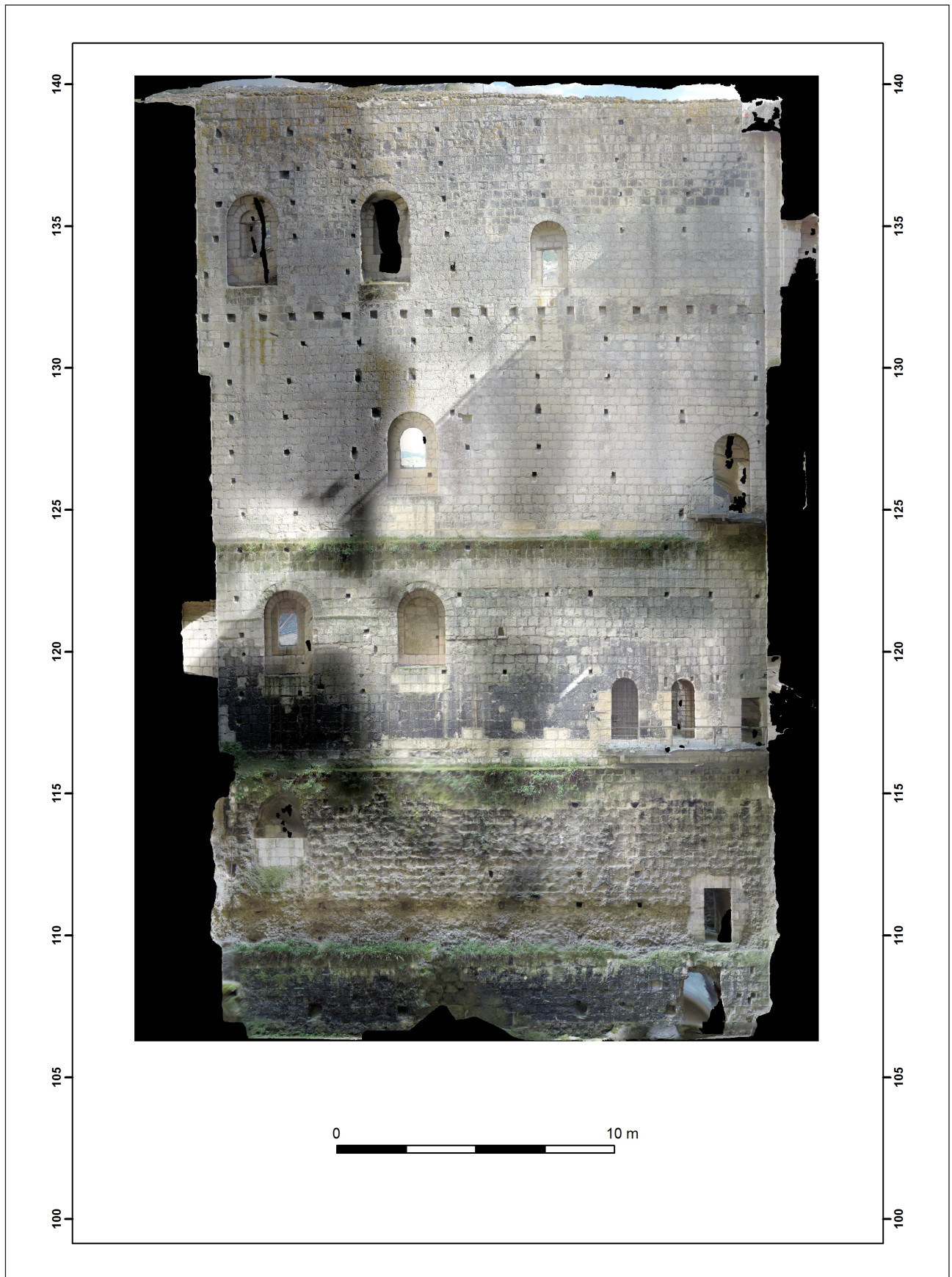
Figure 21 : photogrammétrie de la face interne nord de la grande tour (Pellerin 2017)
