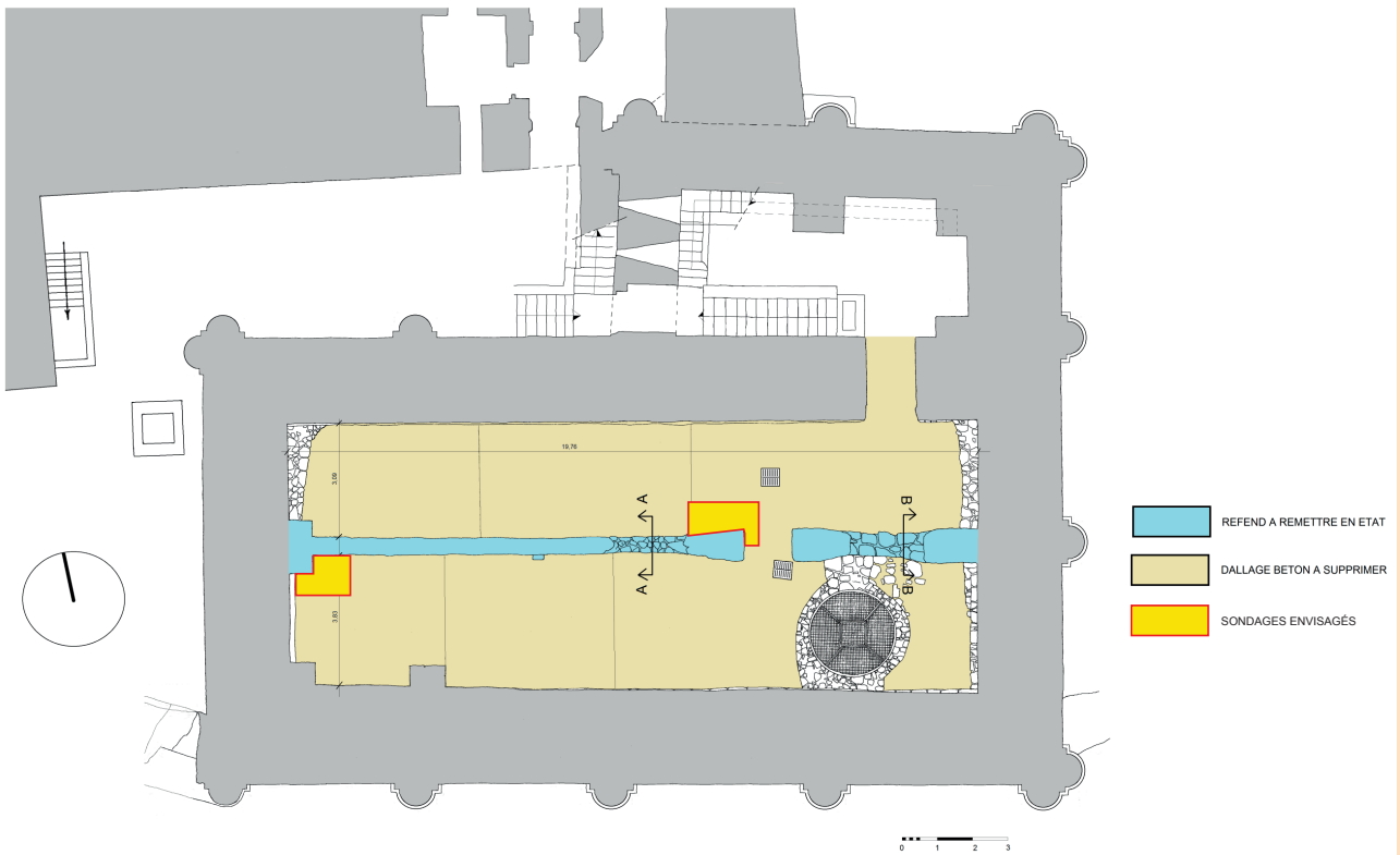
PLAN DE L'IMPLANTATION ENVISAGÉE DES SONDAGES DU DIAGNOSTIC AU DONJON DE LOCHES
