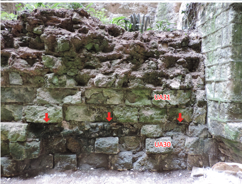
Figure 75 : photographie de détail de la face nord du mur de refend après nettoyage (les flèches indiquent la limite entre les deux phases principales)
