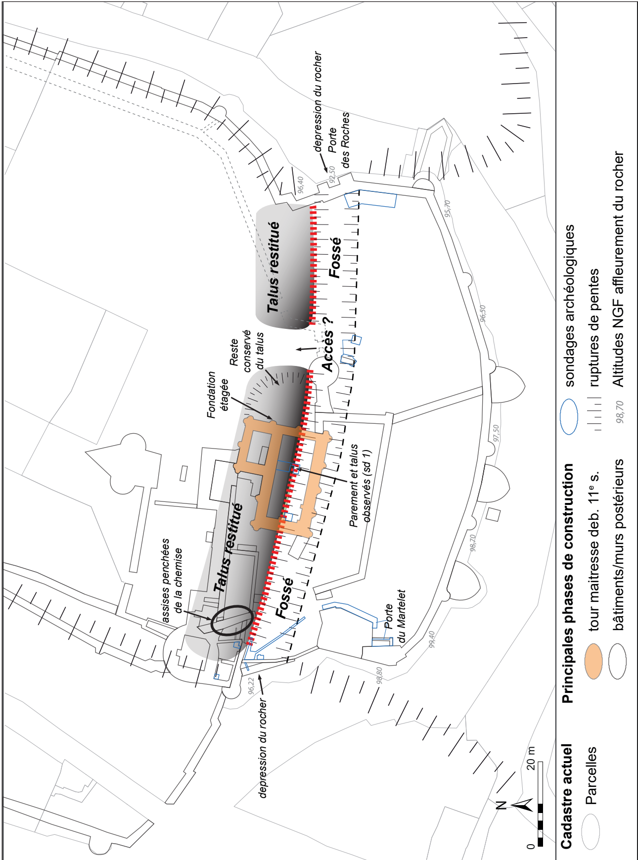
Figure 57 : plan de restitution de l'hypothèse d'un rempart de terre et pierre antérieur à la tour maîtresse
