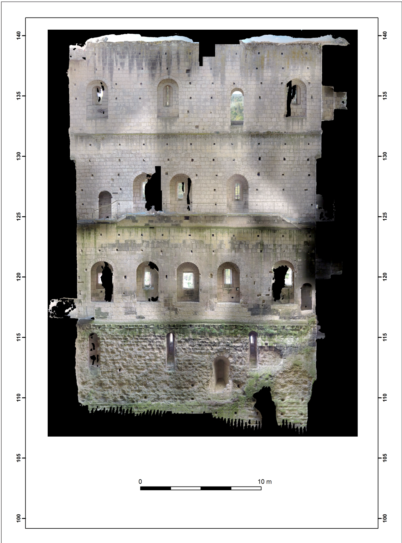
Figure 23 : photogrammétrie de la face interne sud de la grande tour (Pellerin 2017)
