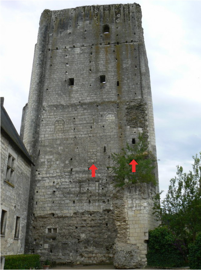
Figure 28 : photographie de la face ouest de la tour maîtresse, avec au premier niveau, les deux portes d'origine bouchées (flèches)
