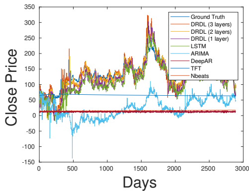
(d) ONGC
