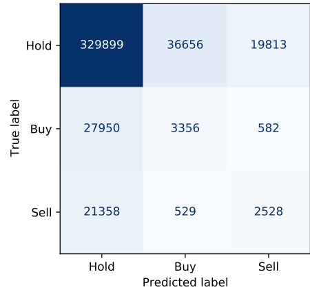
(e) CNN-TA
