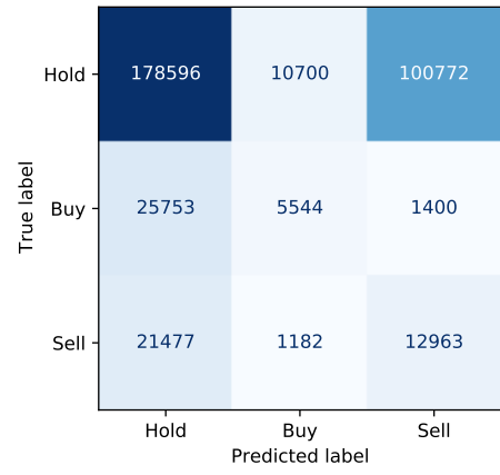
(d) MFNN
