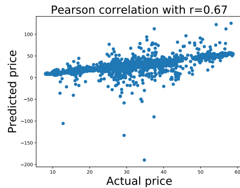
(d) ANF
