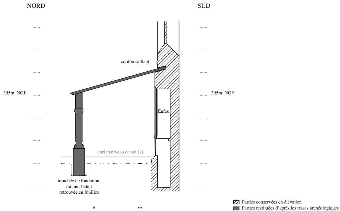
Figure 8 : Restitution du profil de la galerie sud du cloître ; Document Archeodunum SAS.
