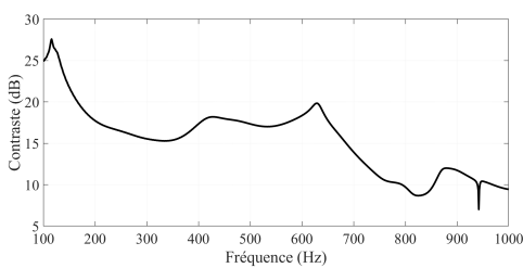
FIGURE 3 – Contraste en statique en fonction de la fréquence
