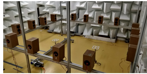
FIGURE 9 – Dispositif expérimental
