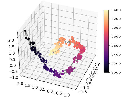
(d) f_3 trajectory corresponding to \mathcal{D}_3 .
