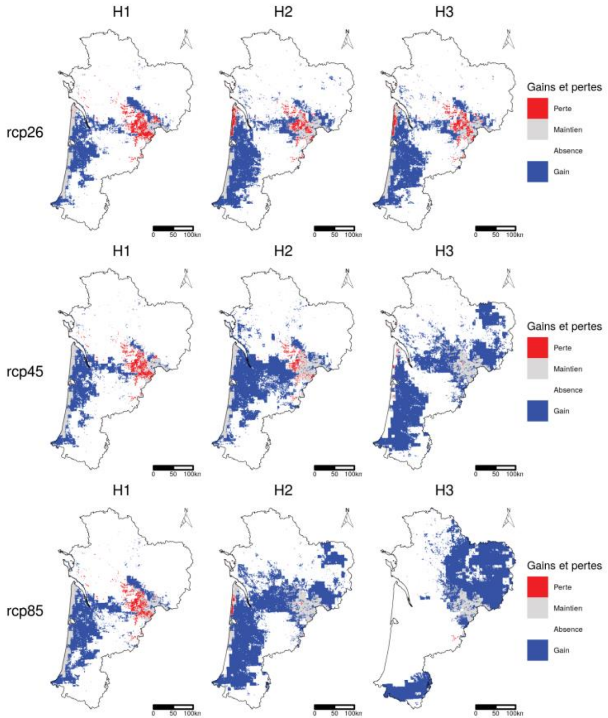
Fig. 172. Changements de la répartition du Léopard ocellé en Nouvelle-Aquitaine, selon la méthode d'ensemble moyenne pondérée. Pourcentages de perte, de gain et de changement total selon les scénarios RCP 2.6, 4.5 et 8.5 aux horizons proche, moyen et lointain.
