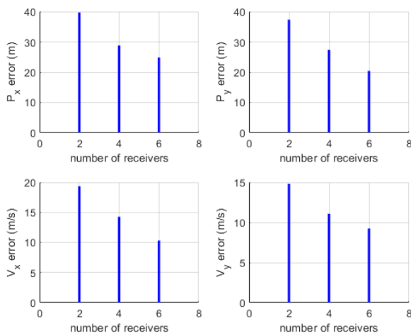
Fig. 4. Error of target parameters estimation.
