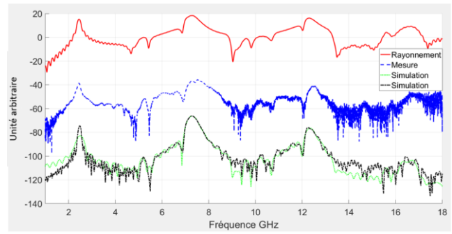
Fig. 6 Comparaison des signaux obtenus : en transmission rayonnée ou champ rayonné -S_{21} , en haut simulé (rouge), au milieu mesuré (bleu) et en bas les champs re-rayonnés (diffracté) lié au mode antenne (noir CC, vert CO).
