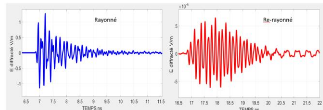
Fig. 5 : Comparaison entre le champ rayonné (mode rayonnement standard) et le champ diffracté (re-rayonné) lié au mode antenne.
