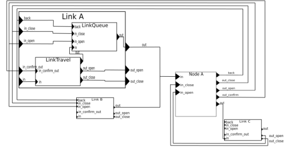
FIGURE 4 – Modèles atomiques à l'échelle mésoscopique.
