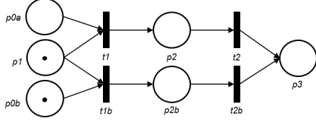
Fig. 3. Petri Net N2
