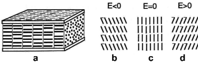
Figure 4 : (a) Smectique A chiral dont les plans des couches sont perpendiculaires aux surfaces de la cellule d'étude. Le champ est perpendiculaire aux surfaces. Vues en surface : (b) Un champ -\vec{E} induit une inclinaison -\theta des molécules. (c) A champ nul. (d) A l'alternance +\vec{E} , une inclinaison +\theta est produite.
