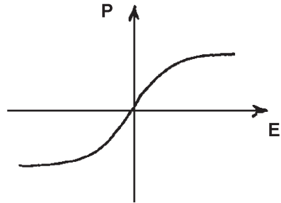
Figure 5 : Variation de la polarisation en fonction de l'amplitude du champ électrique due à l'effet électroclinique dans un smectique A chiral.
