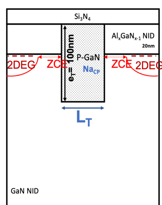
Cellule de base pour la simulation 2D Sentaurus TCAD
