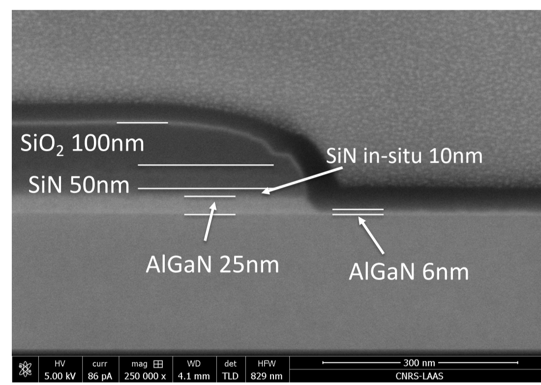
Gravure Cl 2 de l'AlGa N de grille (recessed gate) v = 0,6 nm/s sur wafer 4 pouces
