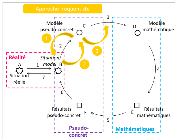
Figure 11. Place de l'approche fréquentiste dans le cycle de modélisation
