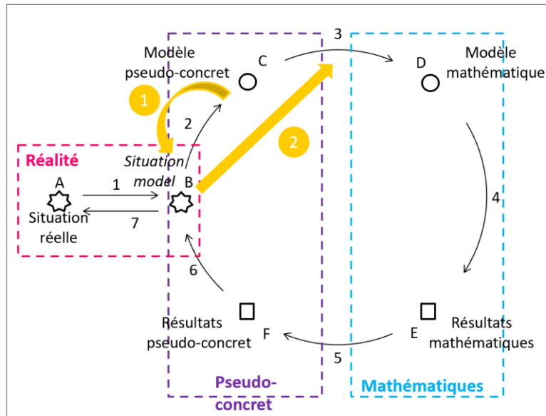
Figure 9. Approche laplacienne : des données statistiques réelles contrôlées par le modèle pseudo-concret
