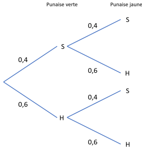
Figure 6. Arbre de probabilité
