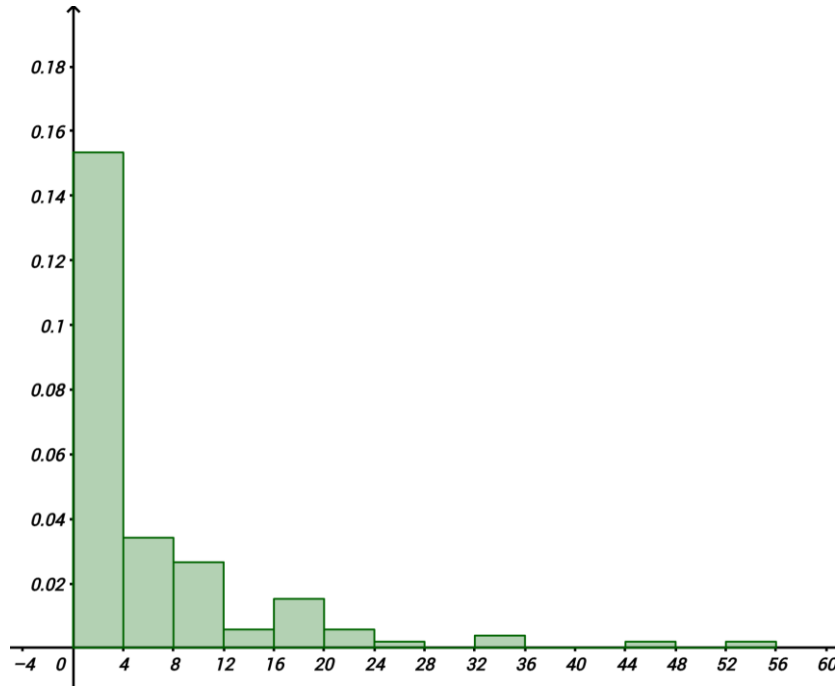
Figure 7. Histogramme des temps d'attente entre deux éruptions consécutives
