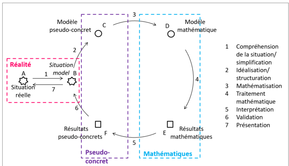
Figure 2. Cycle de modélisation retenu
