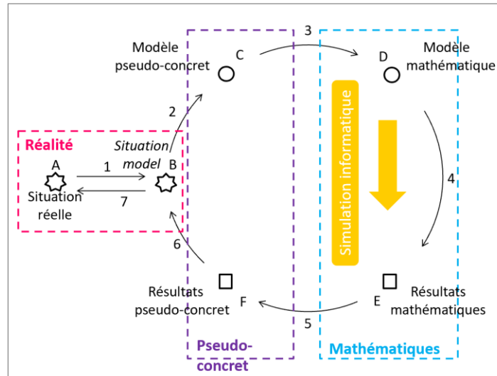
Figure 12. Place de la simulation informatique dans le cycle de modélisation
