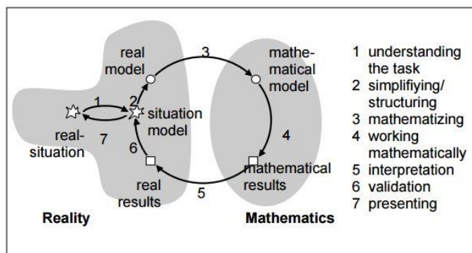
Figure 1. Le cycle de modélisation proposé par Blum et Leiss (2007)
