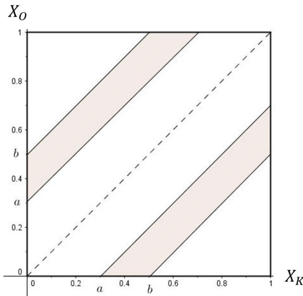
Figure 4. Résolution géométrique (Alory et Derouet, 2018)
