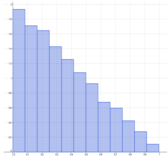
Figure 5. Histogramme d'un échantillon de taille 10 000 avec des classes d'amplitude 5 minutes (Alory et Derouet, 2018)
