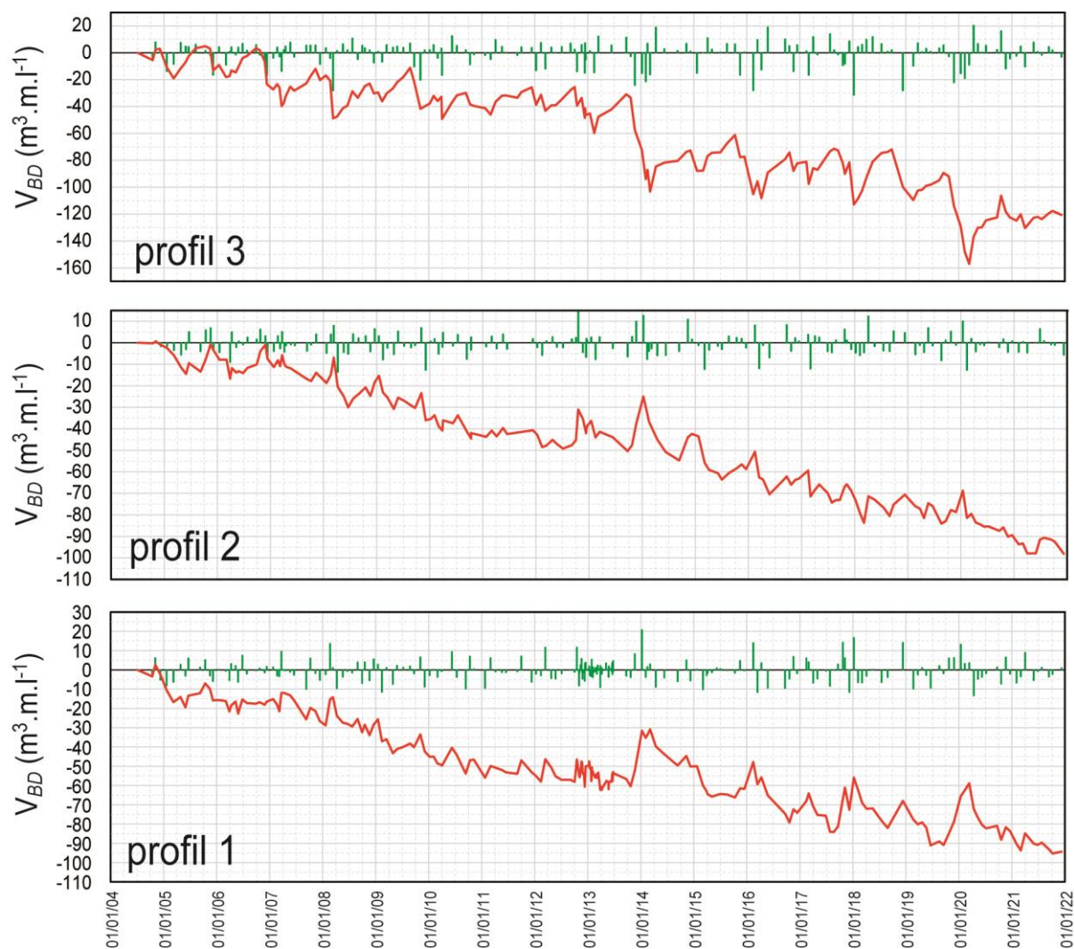
Figure 3 – Bilans sédimentaires du système plage / dune pour les 3 radiales 1, 2, et 3 entre juillet 2004 et décembre 2021 (barres vertes : fréquences séparées ; ligne rouge : fréquences cumulées)
